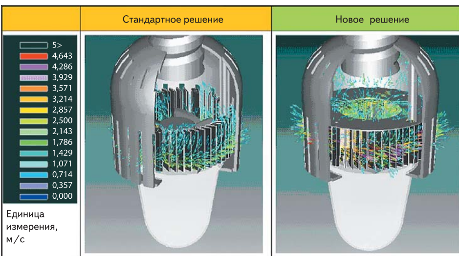
Рис. 2. Сравнение скоростей и направления воздушного потока для стандартного охлаждения и новой модели
