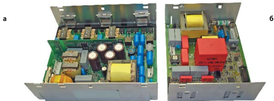
Рис. 3. Драйверы натриевых светильников для переменного (а) и постоянного (б) напряжений питания
