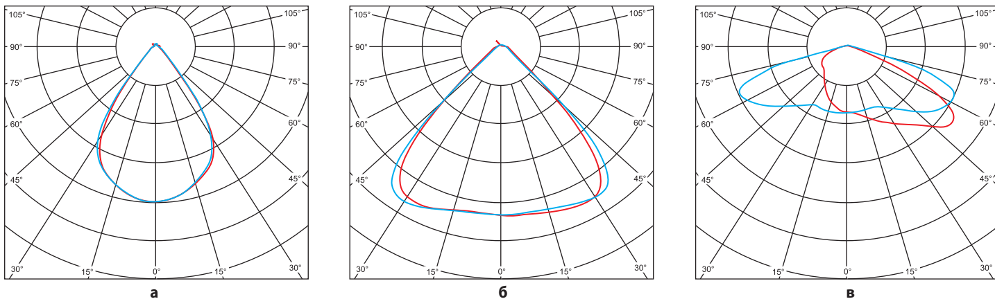
Рис. 5. КСС мультилинз: а) симметричной 60°; б) симметричной 90°; в) широкой боковой 63×154°
