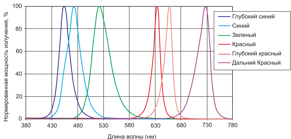
Рис. 7. Спектральные характеристики монохромных светодиодов Cree
