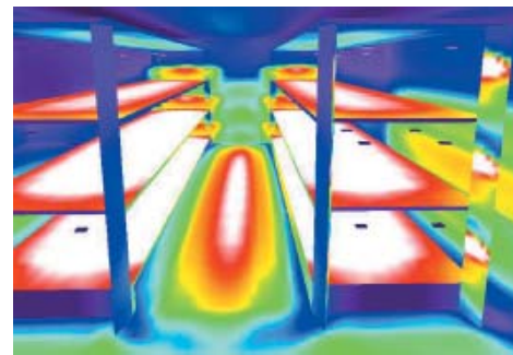
Рис. 17. Освещение стеллажа (результаты расчета E сп = 8080 лк, E мин /E сп = 0,63; PPF D = 149 мкмоль/с/м 2 , ФАР = 26 Вт/м 2 )
