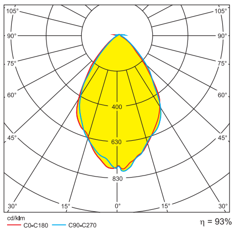
Рис. 15. Диаграмма линзы CS14839_HB-2x2MX-WWW
