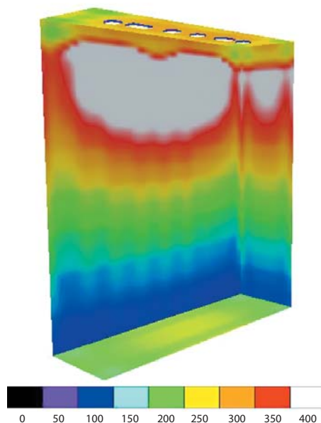
Рис. 20. Распределение освещенности внутри фитотрона (результаты расчета на полу E_{ср} = 11730 лк, E_{мин}/E_{ср} = 0,8 , PPFD = 215 мкмоль/с/м 2 , ФАР = 39 Вт/м 2 )
