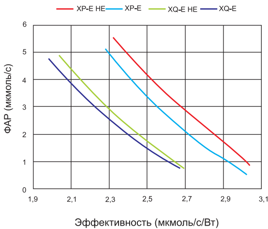
Рис. 8. Характеристики светодиодов XQ-E и XP-E Royal Blue и High Efficacy Photo Red
