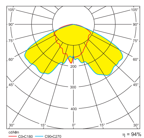
Рис. 19. Диаграмма линзы C14642_FLORENCE-1R-UP
