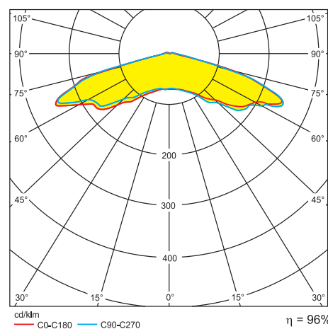
Рис. 18. Диаграмма линзы CS14764_STRADA-2x2MX-VSM
