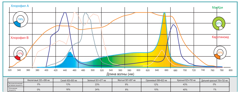
Рис. 11. Спектр излучения Фито Strada_2×2MX&Jenny_4×16_XQE
