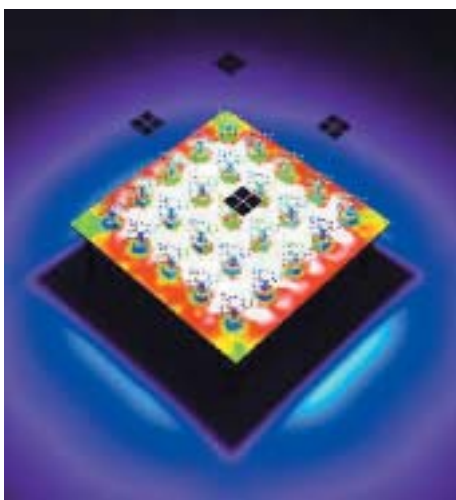
Рис. 16. Освещение растений на столе (результаты расчета E сп = 15340 лк, E мин /E сп = 0,61, PPF D = 281 мкмоль/с/м 2 ; ФАР = 51 Вт/м 2 )
