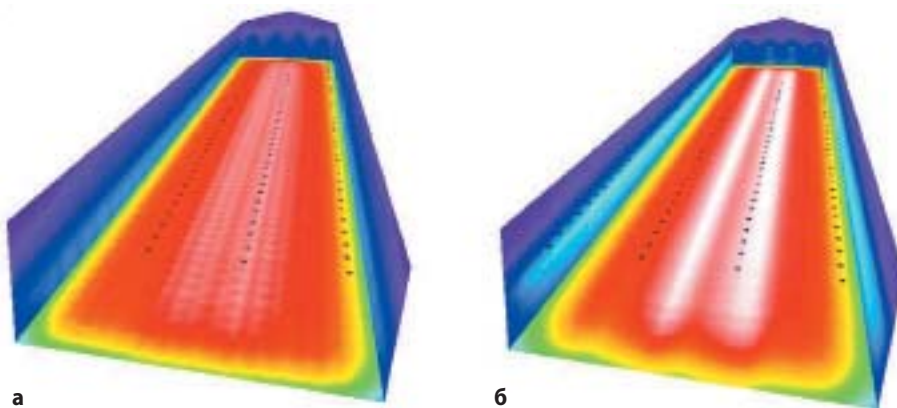
Рис. 14. Освещение теплицы сверху: а) с оптикой CS14713_НВ-2Х2МХ-В с матрицей 4×16_ХQ-Е (Е ср = 4100 (4600) лк, Е мин /Е макс > 0,58, PPFД = 75 (84) мкмоль/с/м 2 , ФАР = 14 (15) Вт/м 2 , СДС (16 ч) = 4,3); б) с оптикой CS14839_НВ-2Х2МХ-WWW с матрицей 4×16_ХQ-Е (Е ср = 4100 (4800) лк, Е мин /Е макс > 0,44, PPFД = 74 (88) мкмоль/с/м 2 , ФАР = 13 (16) Вт/м 2 , СДС (16 ч) = 4,3)
