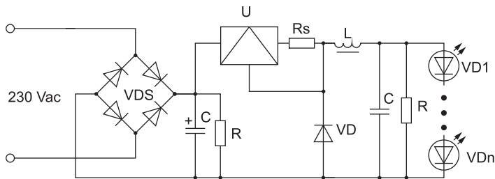
Рис. 10. Типовая схема встроенного импульсного драйвера
