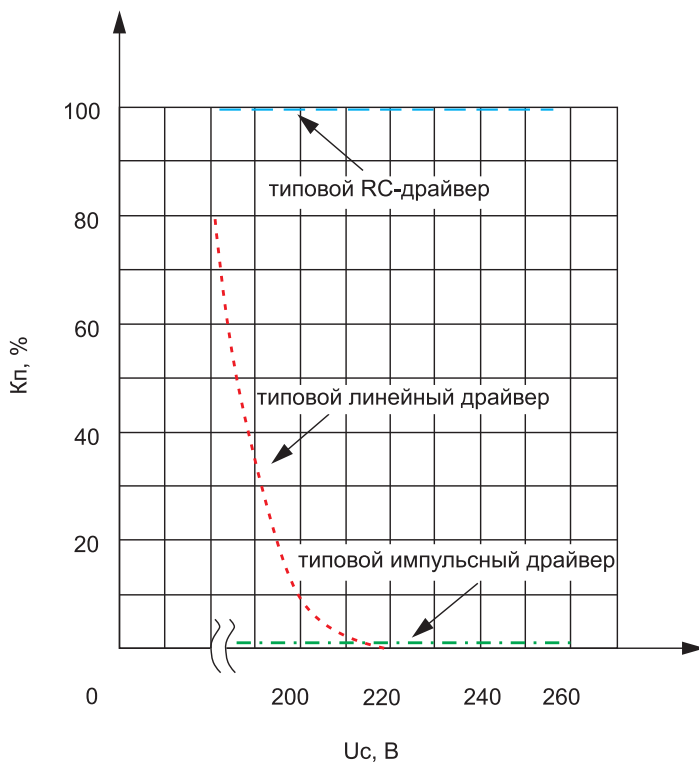
Рис. 12. Зависимость K_{П} типовых СДЛ со встроенными драйверами от напряжения питающей сети
