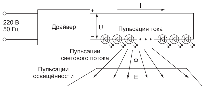
Рис. 5. Обобщенная схема системы освещения
