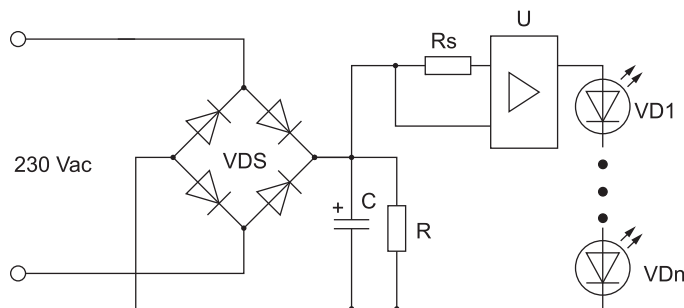
Рис. 8. Типовая схема встроенного линейного драйвера
